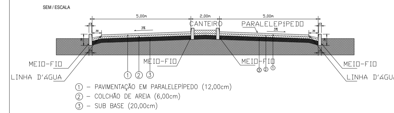
SEÇÃO TRANSVERSAL TIPO DA RUA PAULO VALENTIM SEBASTIANA LUZIA SANTANA COELHO (PARALELEPÍPEDO)
