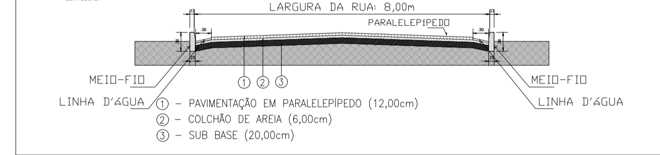
SEÇÃO TRANSVERSAL TIPO DA RUA PAULO VALENTIM SEBASTIANA LUZIA SANTANA COELHO (PARALELEPÍPEDO)
